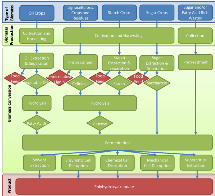
Figura 55 - Cadeias de produção de PHA
